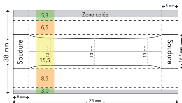
STRUCTURE DE L'EMBALLAGE PAPIER POUR SUCRES MORCEAUX
