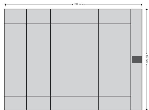
STRUCTURE DE L'EMBALLAGE DES PERLES RONDES
