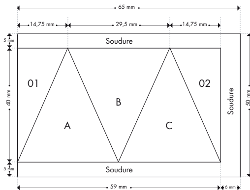
STRUCTURE DU BERLINGOT PAPIER
