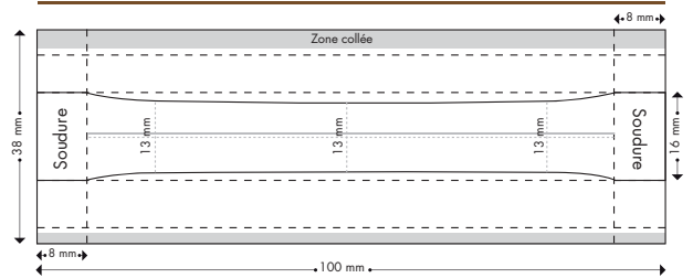
STRUCTURE DES BÛCHETTES TRANSPARENTES
